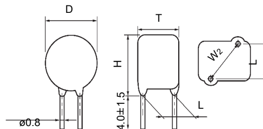
(ERZV10D182CS)
