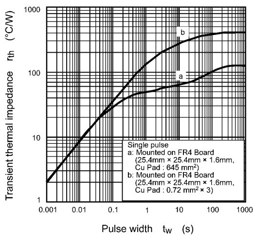
Fig. 7.12 r_{th} - t_w
